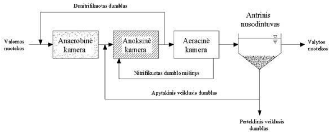
2 pav. Klaipėdos miesto nuotekų valyklos biologinio valymo technologinė schema.
