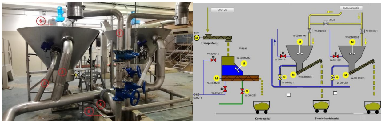
8 pav. Smėlio separatorius
