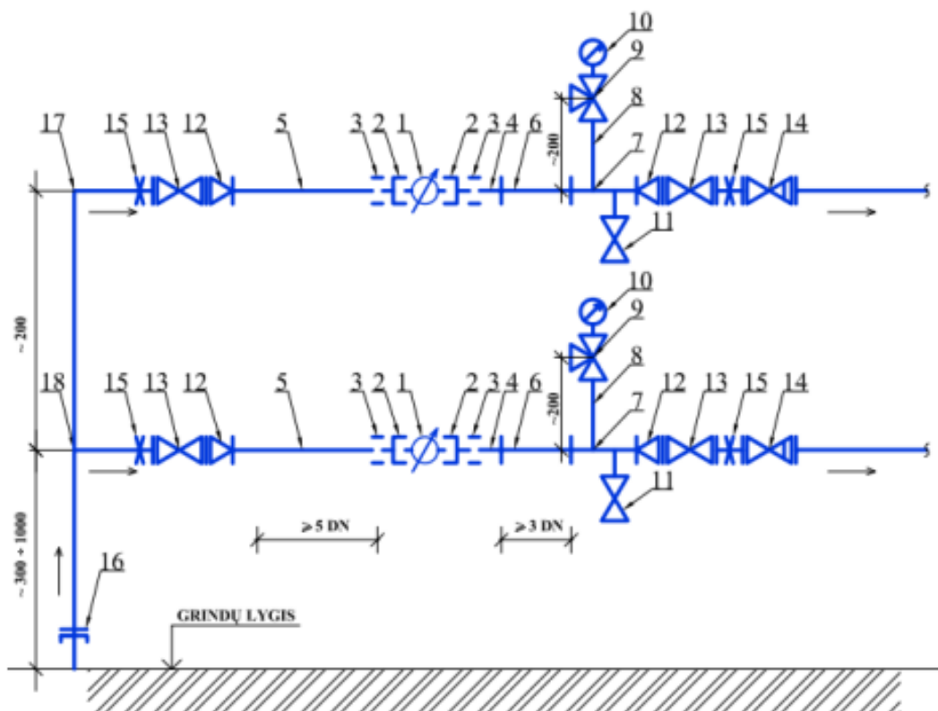
Lygiagretaus vandens paskaitos mazgo montavimo schema
