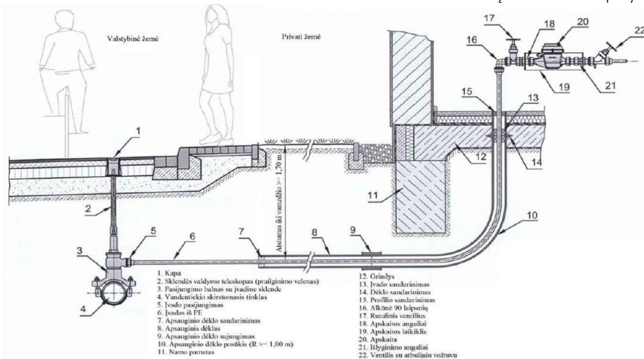
Schema Nr. 2 Vandentiekio įvado trasavimo pavyzdys
