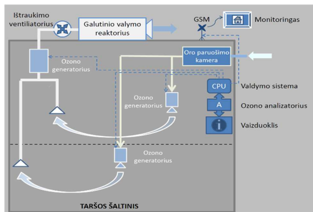
6 pav. Pirmoji Lietuvoje automatinė kvapų neutralizavimo ozonu sistema
