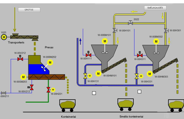
8 pav. Smėlio separatorius
